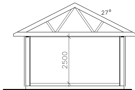
SCHNITT ANBAU
