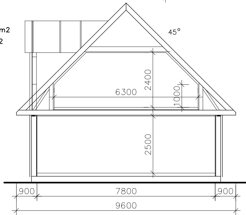
SCHNITT
